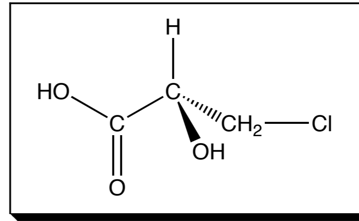
光学異性体 (鏡像異性体)
